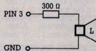
Bild 6. Lautsprecheranschluß
